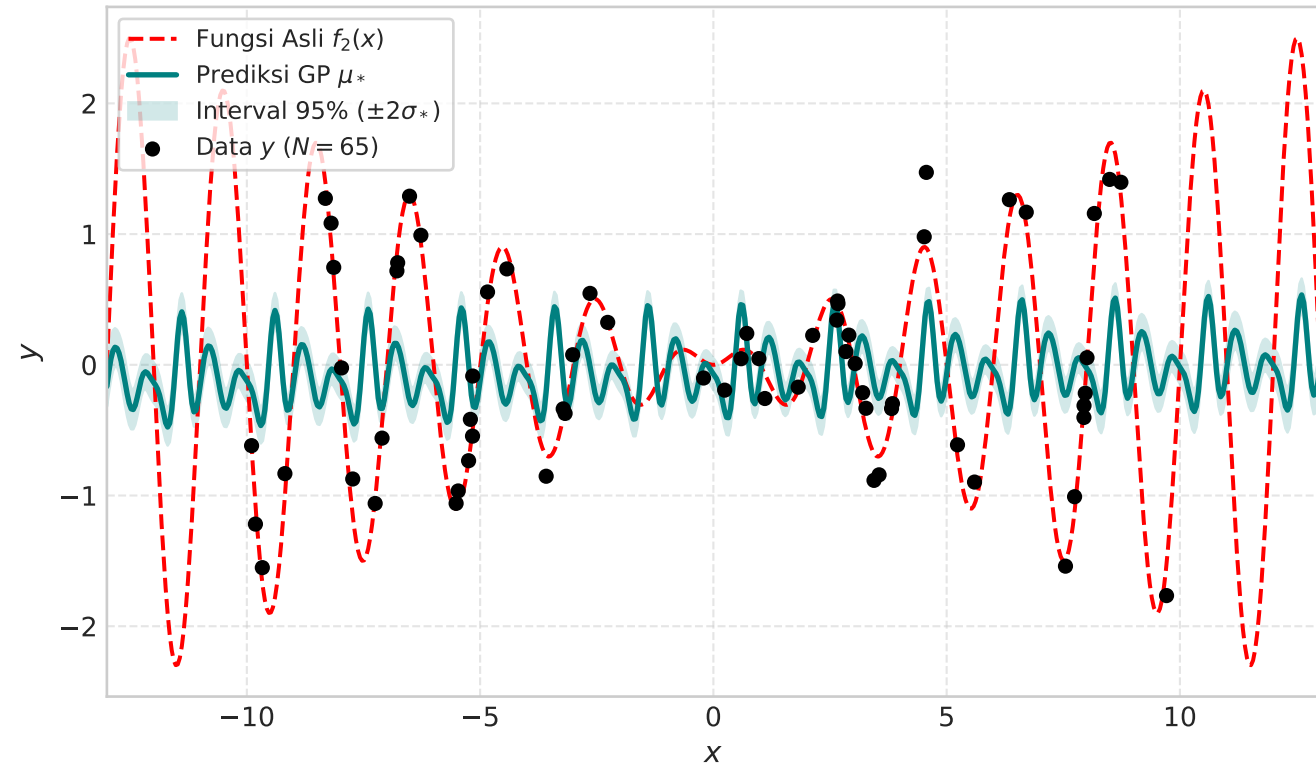
(a) Penjumlahan: k_{\text{Lin}} + k_{\text{Per}}
